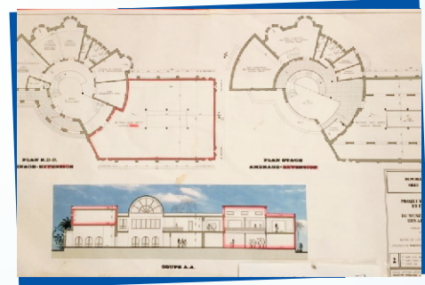
Plan d'extension
